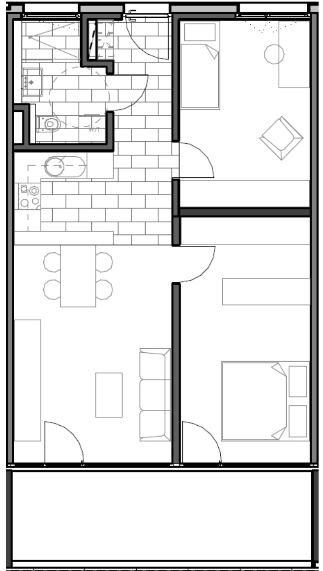
Grundriss 3.5 Zimmer
